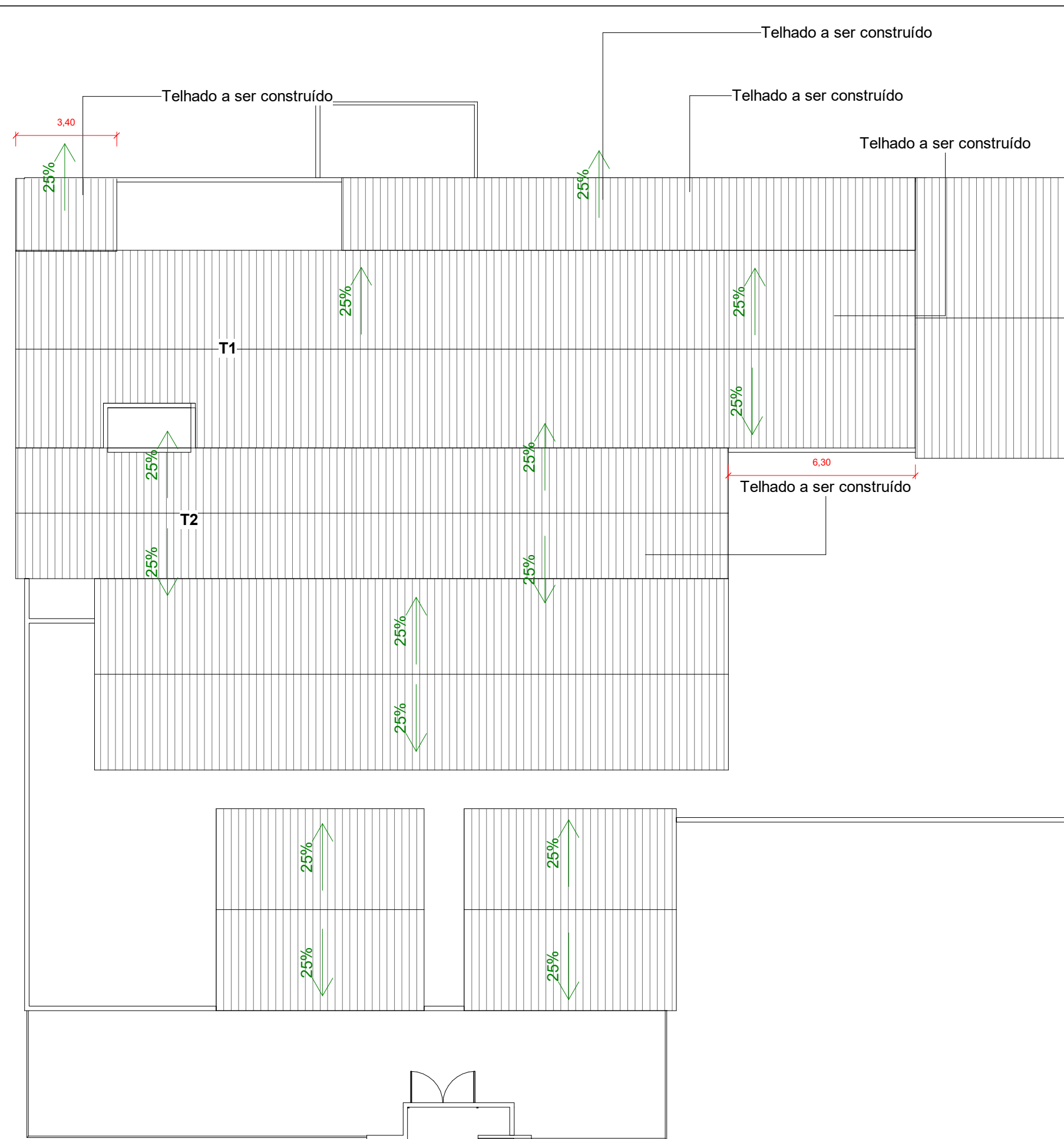
6 Vista de Cobertura - Resultado
