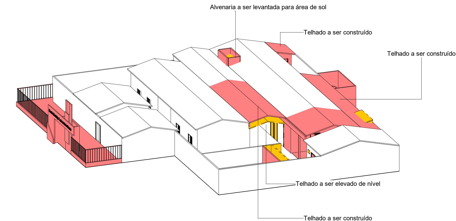
12 3D - DETALHE SOBRE OS TELHADOS
