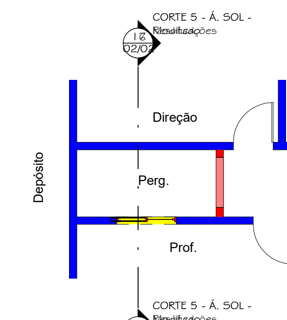
18 Detalhe - Área de Sol - Modificações
