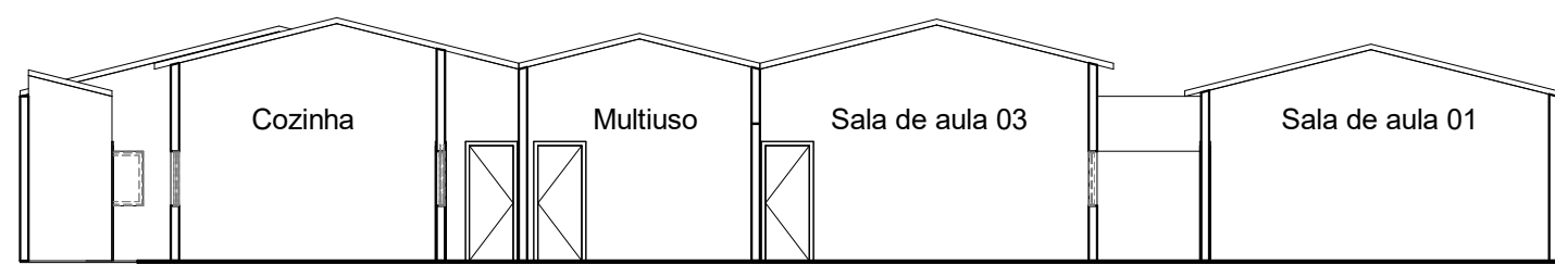
8 CORTE 1 - ANTES DA REFORMA 1 : 150
