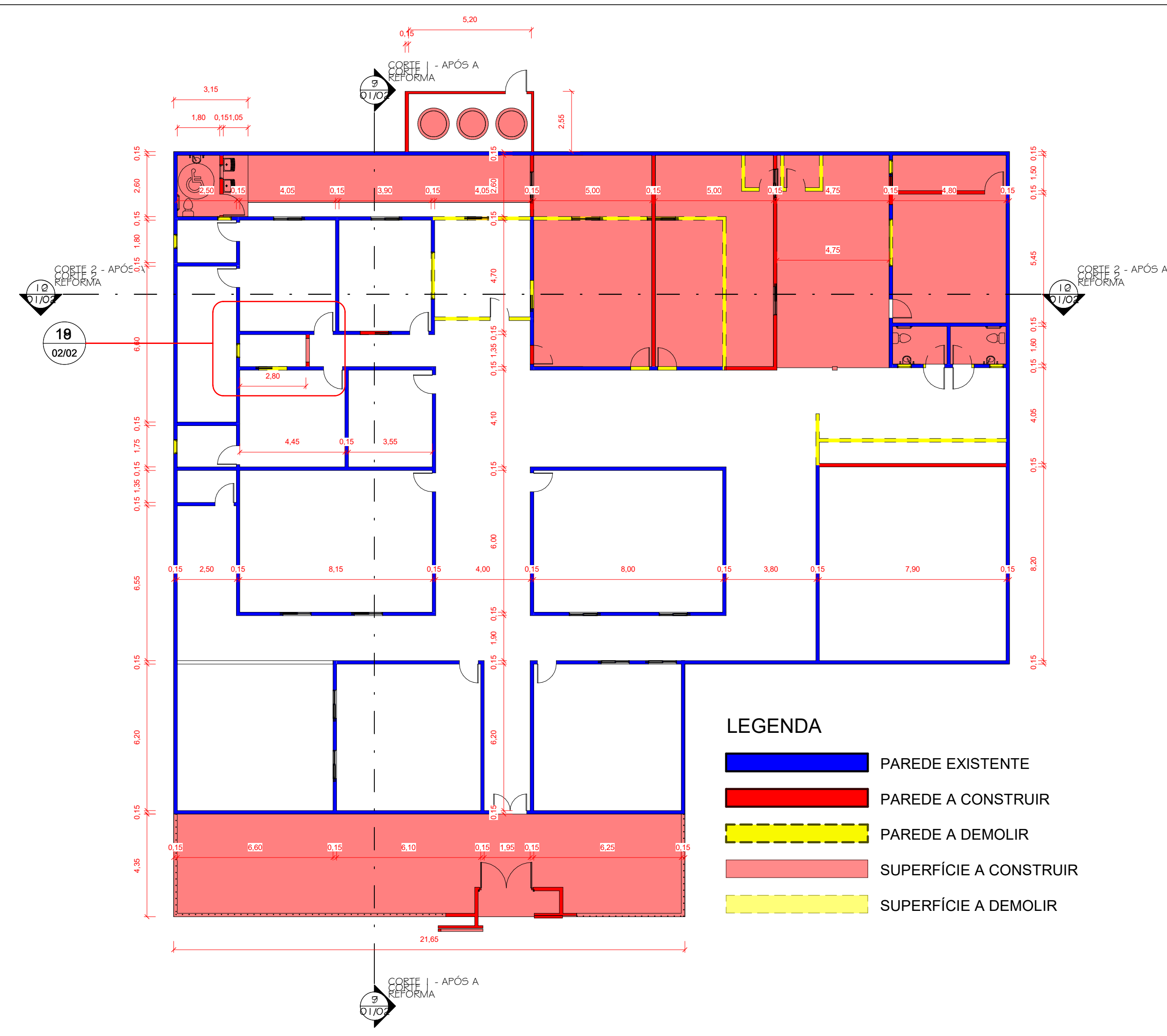
2 Pav. Térreo - Modificações 1 : 150
