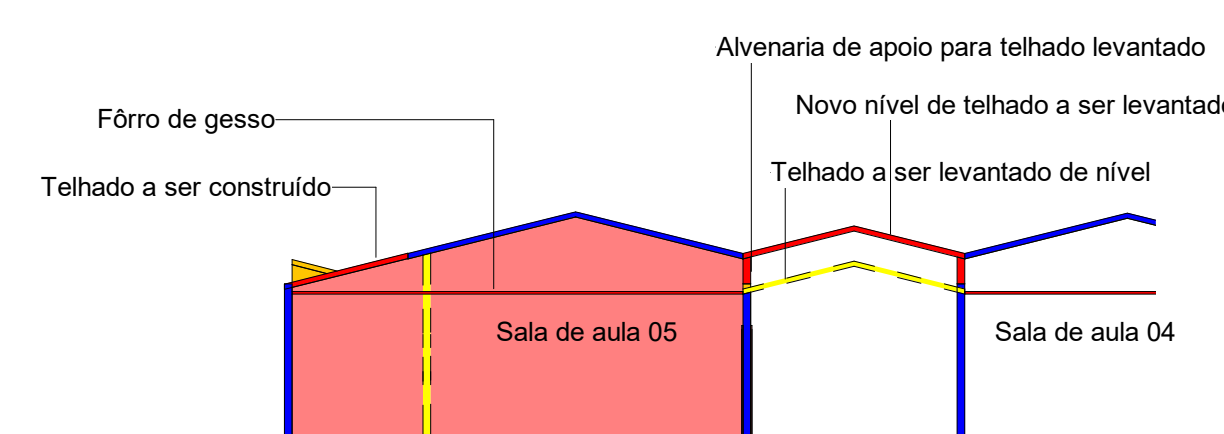
4 CORTE 3 - Novas salas - Modificações
