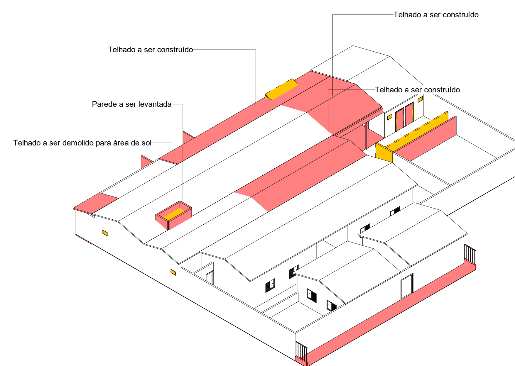
13 3D - DETALHE SOBRE OS TELHADOS - SEGUNDA VISTA
