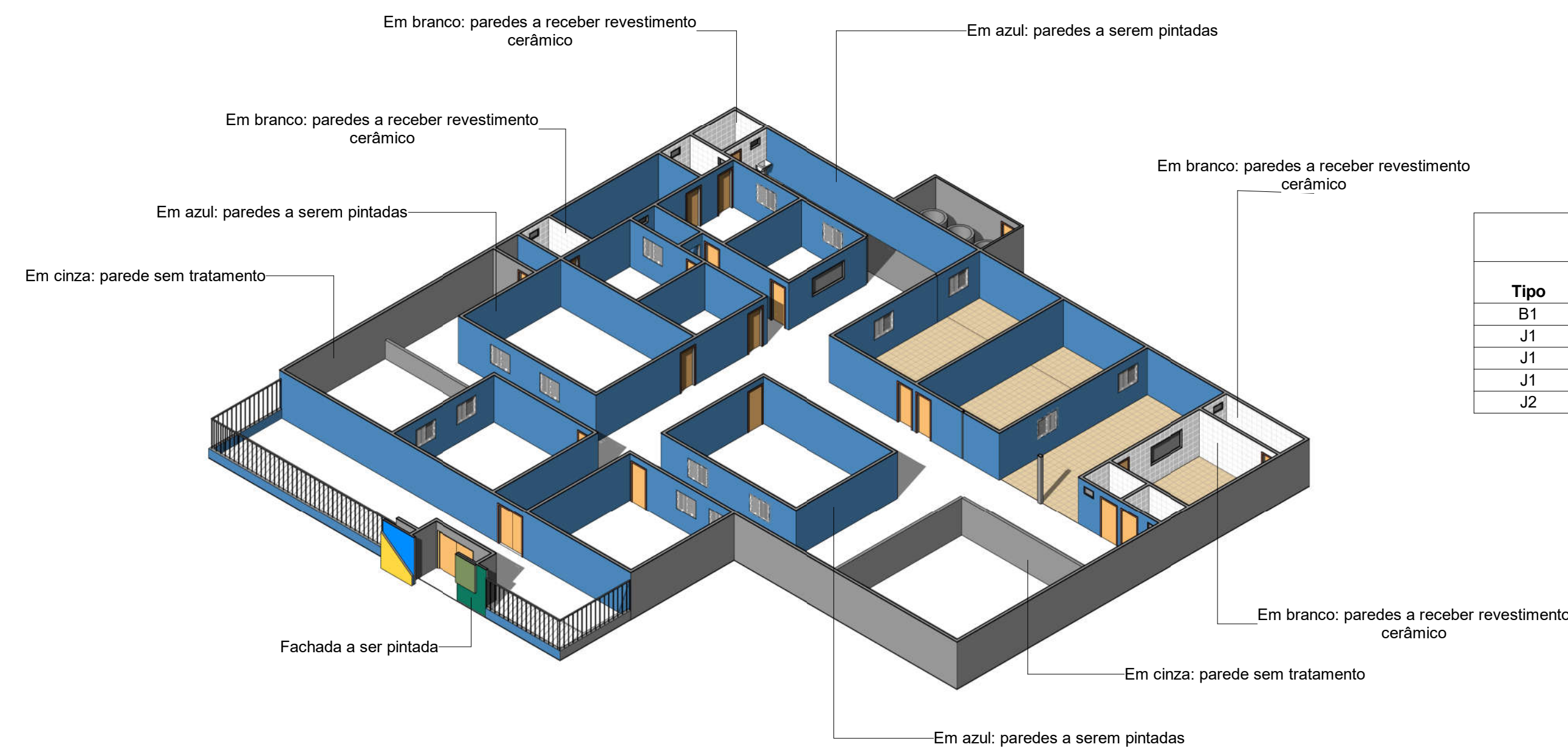
13 3D - Tratamento em paredes (com corte)
