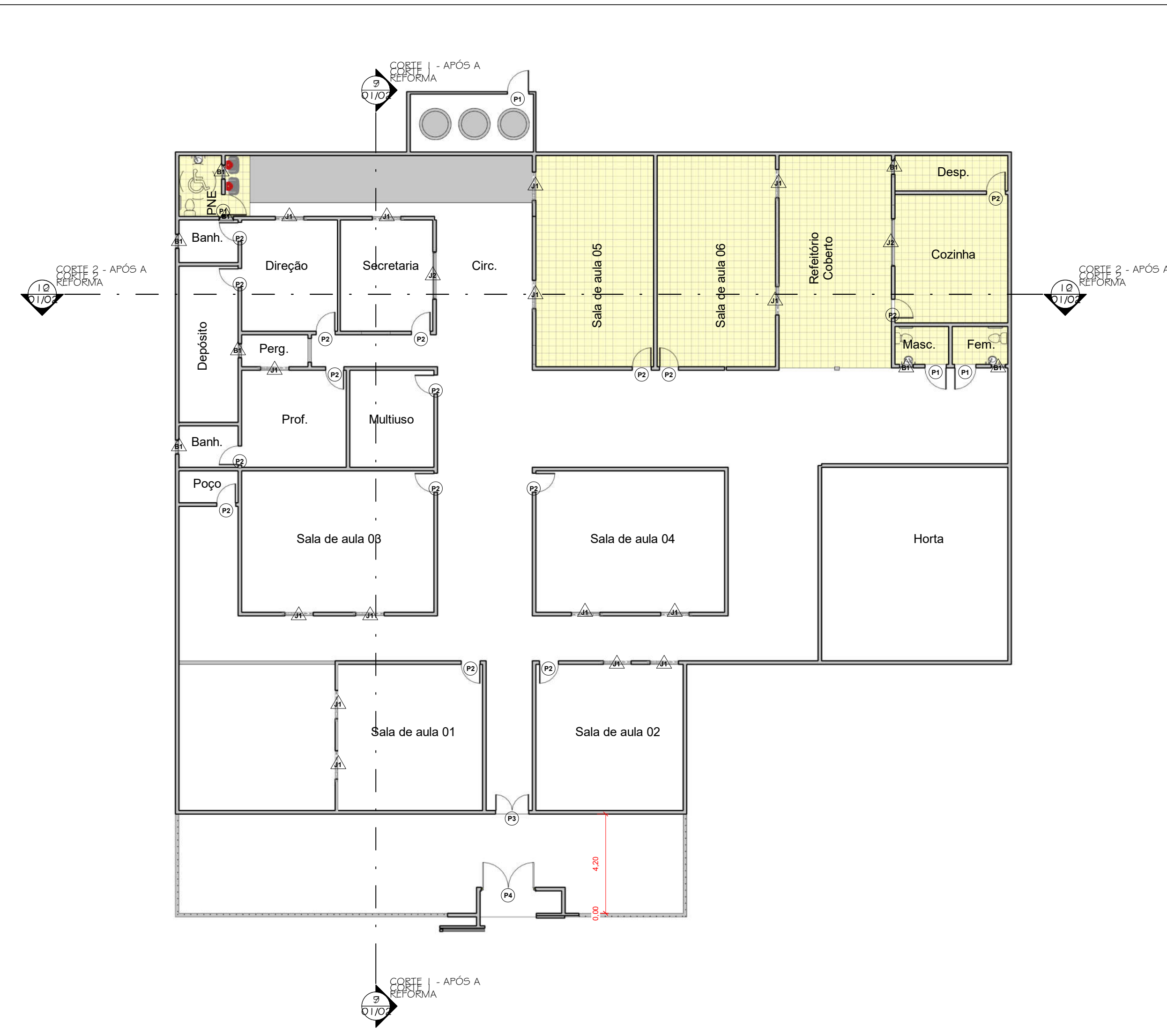
3 Pav. Térreo - Resultado final 1 : 150
