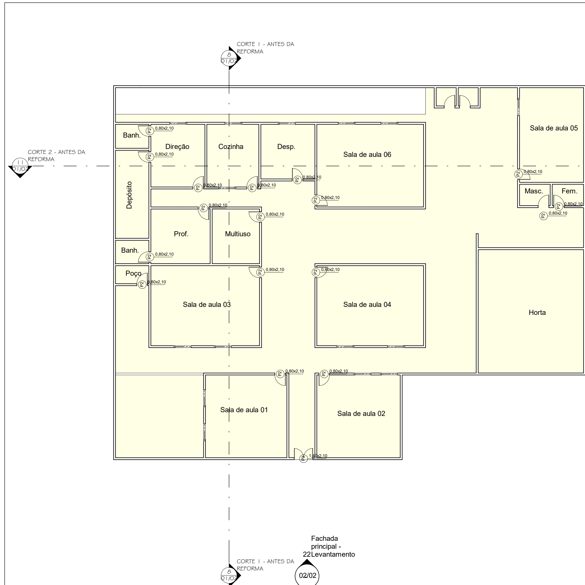
1 Pav. Térreo - Levantamento 1 : 150
