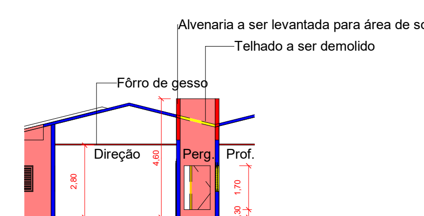
16 CORTE 5 - À. SOL - Modificações
