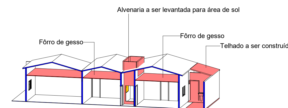
14 3D - DETALHE - ÁREA DE SOL - Modificações
