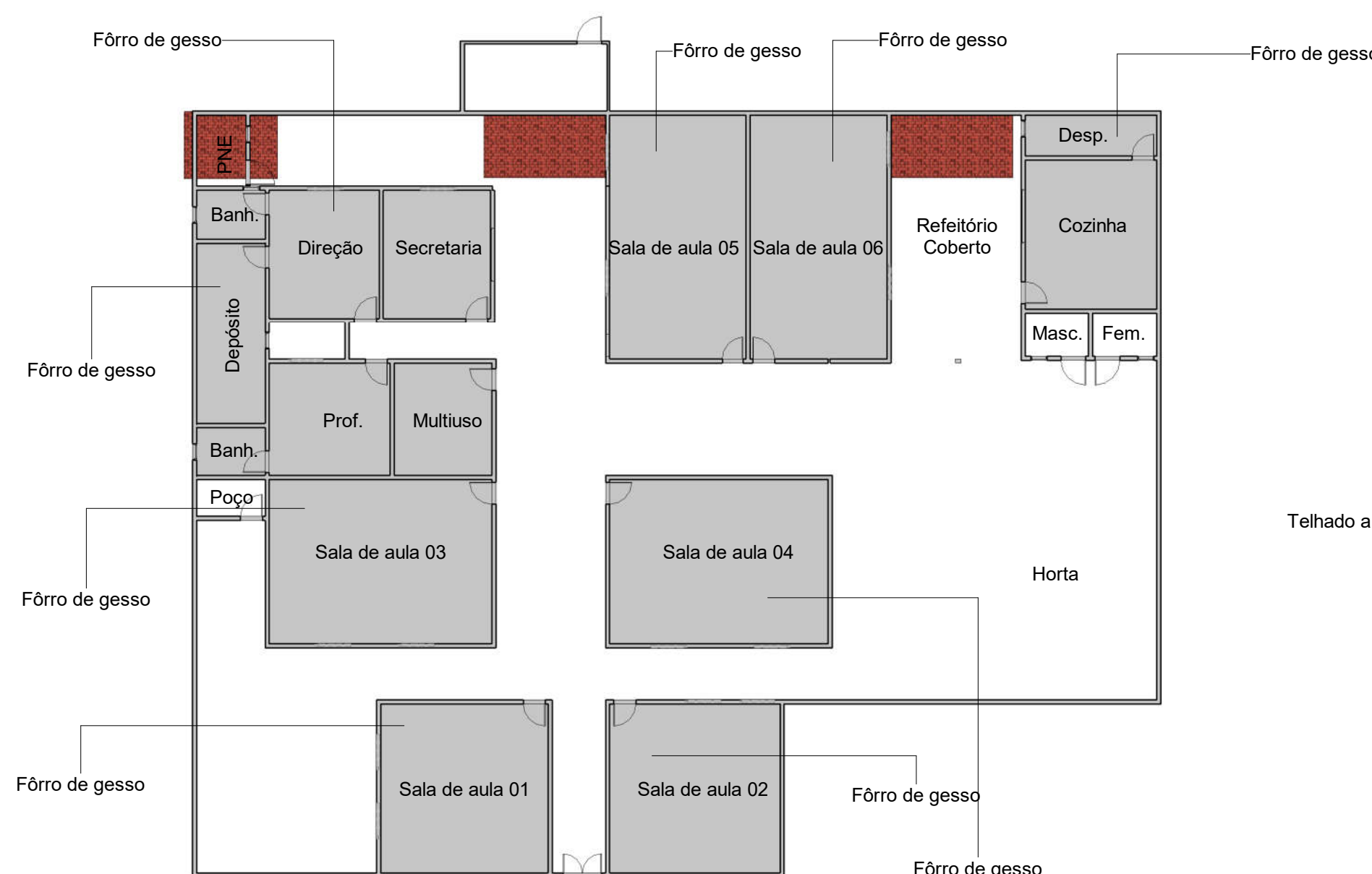
7 Planta de fôro (vista de baixo para cima)
